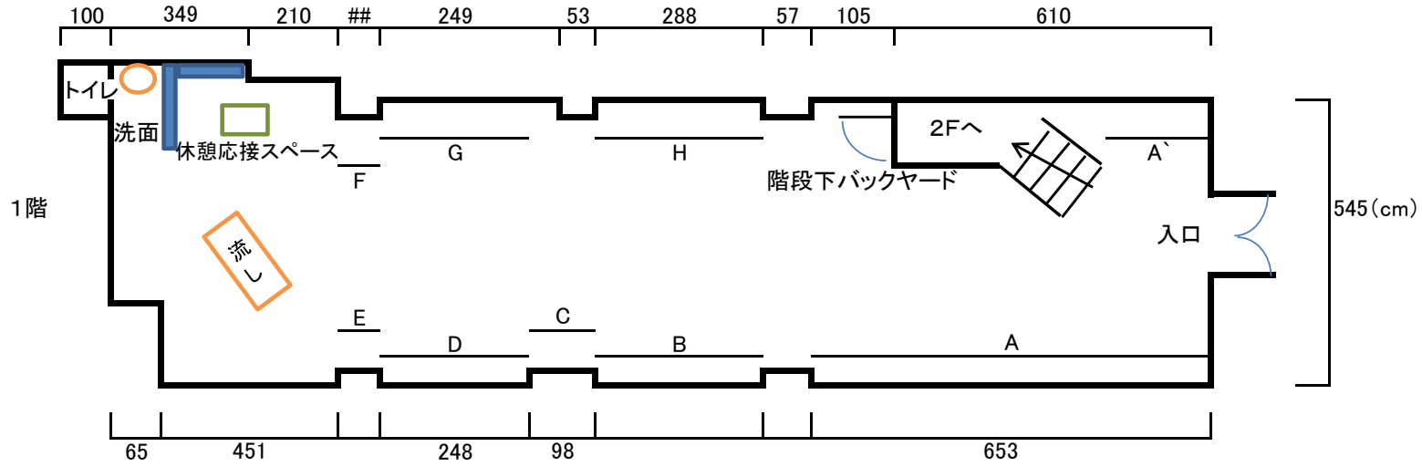
大手筋ギャラリー見取り図概観 (単位はcm)
